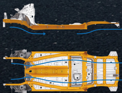
โครงสร้างช่วงล่างจากเหล็ก High-tensile เชื่อมต่อกันอย่างสมบูรณ์แบบ ให้ความแข็งแรง ปลอดภัยในทุกการขับขี่ และประหยัดน้ำมันมากขึ้น
